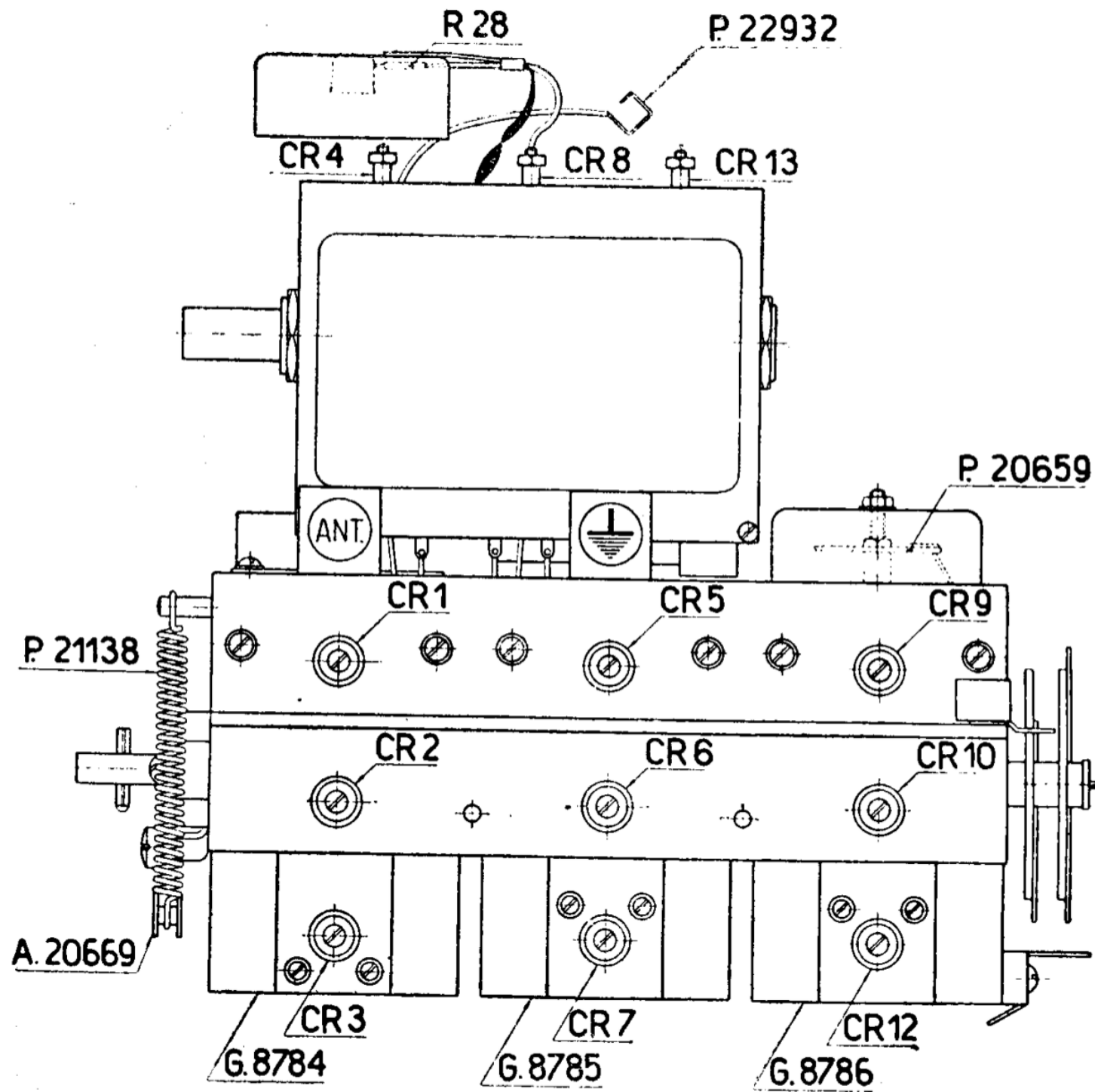
Il castello AF del mod. « 543 » Safar.
